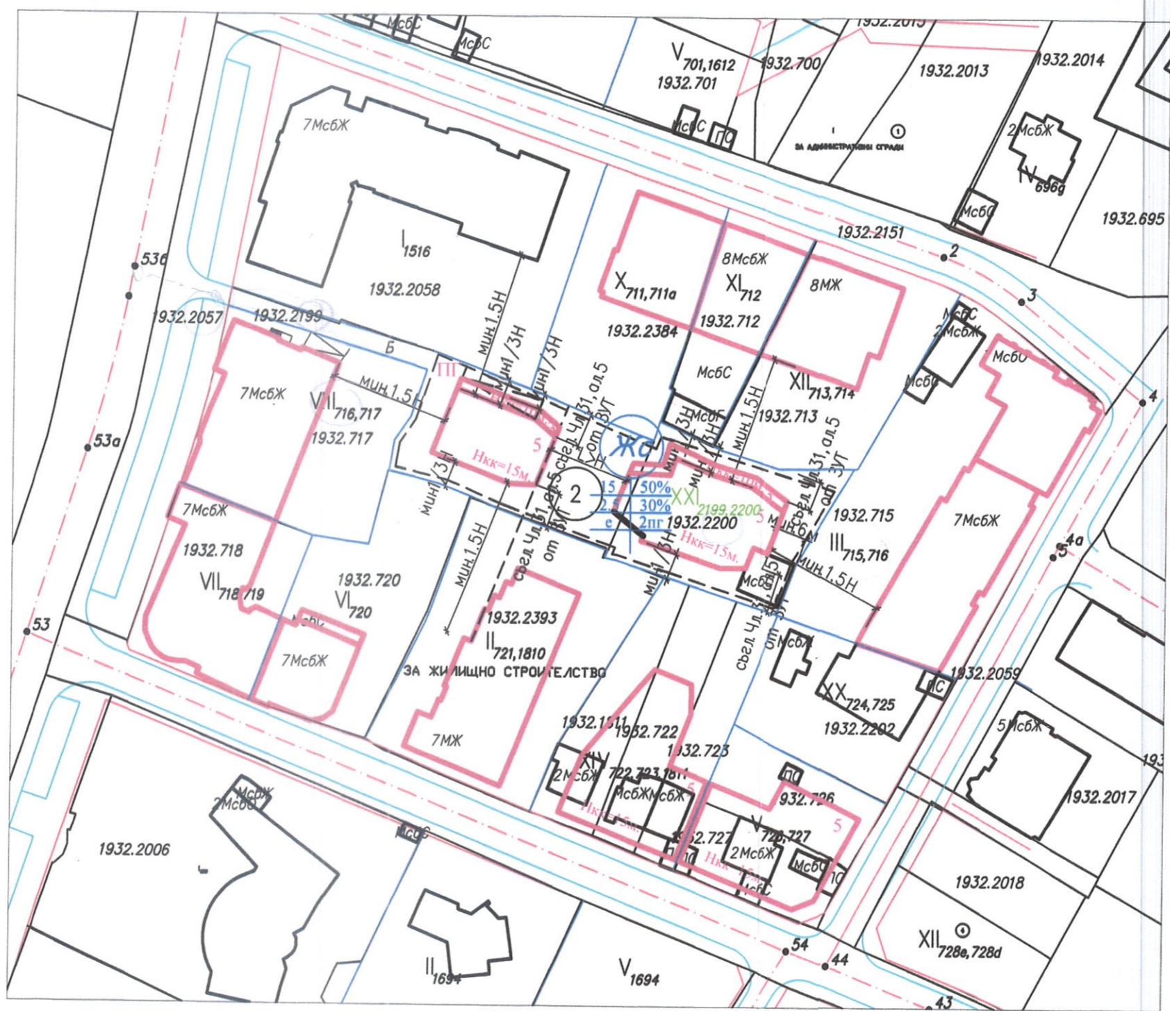
МОТИВИРАНО ПРЕДЛОЖЕНИЕ ЗА ИЗМЕНЕНИЕ НА ЗАСТРОИТЕЛЕН ПЛАН М 1:1000
